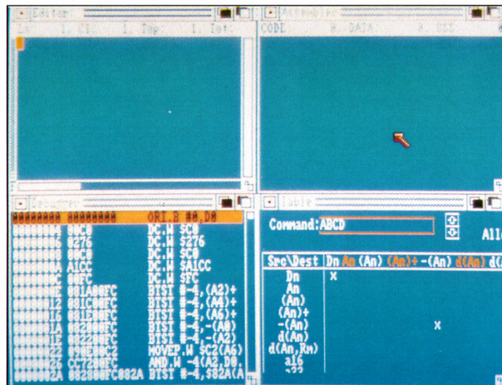
AssemPro er opbygget med disse 4 vinduer
